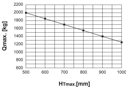
Abb. 12a Beispiele für die größte Gefachhöhe HTmax. Exemple de hauteur de compartiment maximale HTmax. Voorbeelden voor de grootste vakhoogte HTmax. Examples for the largest shelf height HTmax.
