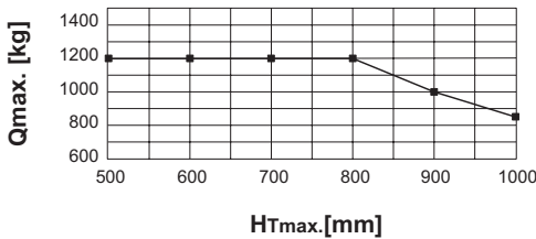
Feldlasten für Regalhöhe 2500 und 3000 mm Charges de travée pour des hauteurs d'étagère comprises entre 2500 et 3000 mm Veldbelastingen voor stellinghoogtes 2500 en 3000 mm Bay loads for a rack height of 2500 and 3000 mm
